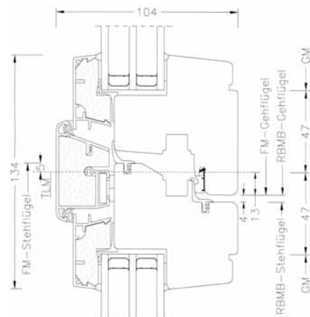
Schnitt Stulp
