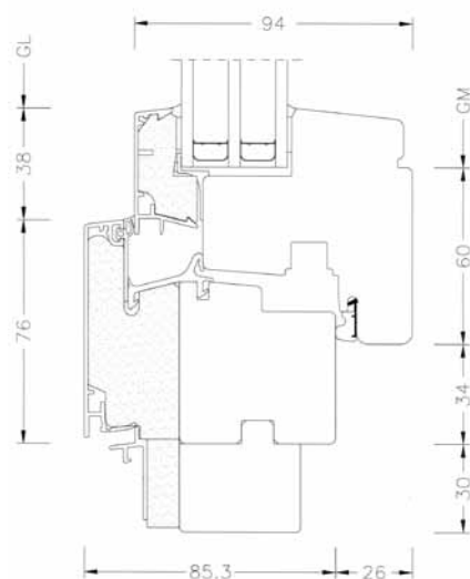
Schnitt senkrecht
